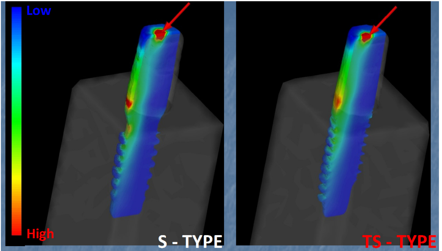
500N 荷重時インプラント周囲骨応力解析 圧縮応力 (MPa)
