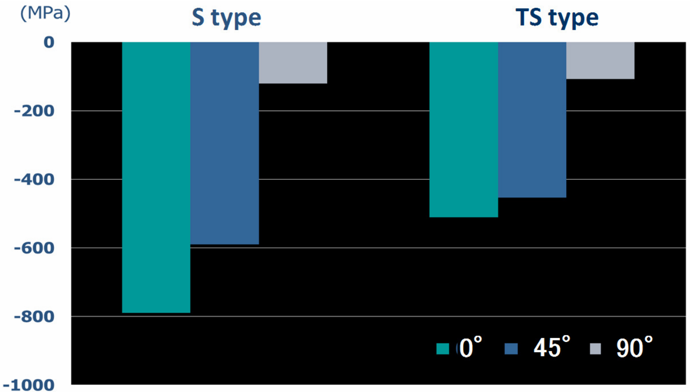
500N 荷重時インプラント周囲骨応力解析 圧縮応力(再小主応力) (MPa)
